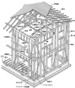
▲一般的な木造住宅の軸組
